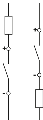
Esquema de conexiones DLS 6hdc, característica B, un polo
