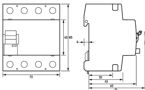
Dibujo acotado Interruptores-seccionadores DHS 4-080 R
