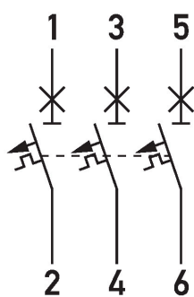
Anschlussschema
