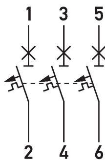
Anschlussschema DLS 6i, B-Charakteristik, dreipolig, 6kA
