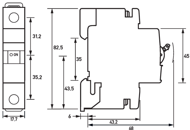
Maßzeichnung DLS 6i, B-Charakteristik, einpolig, 6kA (Gruppenansicht)
