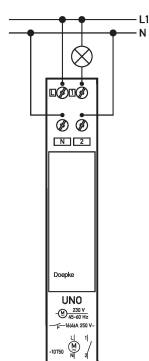
Ejemplo de cableado Relojes programadores Uno QRD
