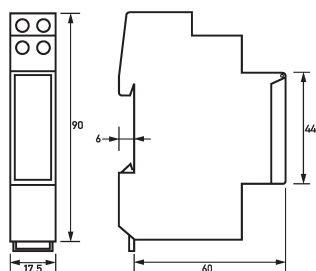
Dibujo acotado Relojes programadores Uno QRD
