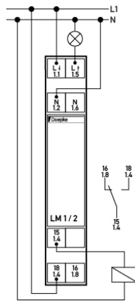
Schaltungsbeispiel
