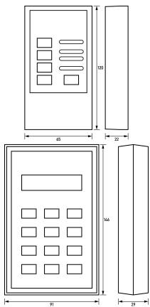
Dibujo acotado Vista de grupos
