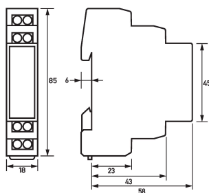
Maßzeichnung Stromstoßschalter (Fernschalter) SIR
