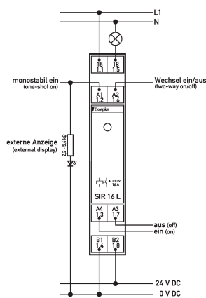
Schaltungsbeispiel Stromstoßschalter (Fernschalter) SIR
