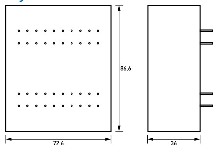
Maßzeichnung Gruppenansicht
