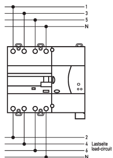
Ejemplo de cableado Interruptores diferenciales DRCCB 5 STR 025-4/0,03-A
