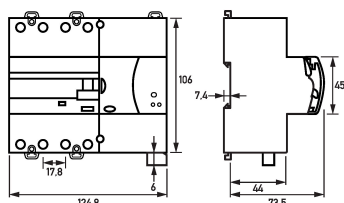
Dibujos acotados Interruptores diferenciales DRCCB 5 STR 025-4/0,03-A
