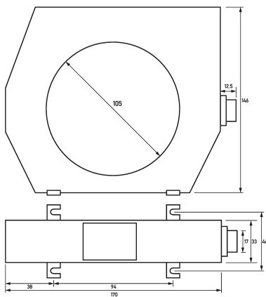
Dibujo acotado Vista de grupos
