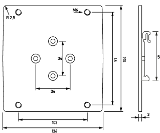
Dibujo acotado Vista de grupos
