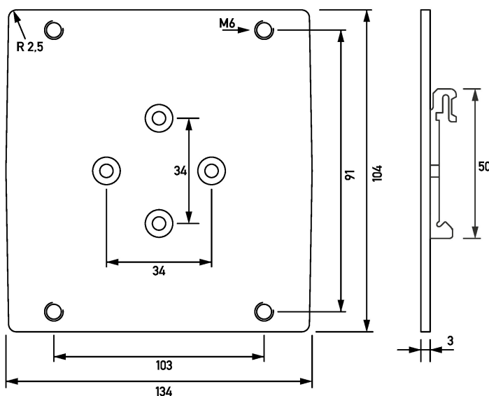
Maßzeichnung RCM Mount B (Gruppenansicht)
