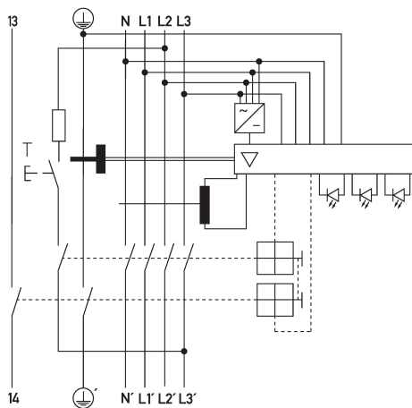
Anschlussschema DPRCD-M+
