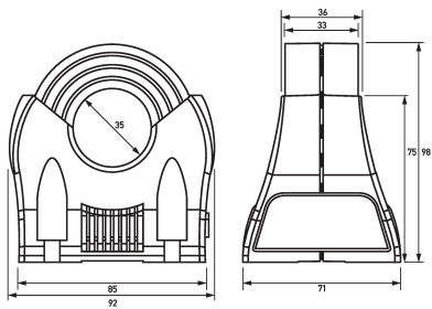
Dibujo acotado Vista de grupos
