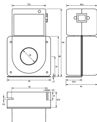
Maßzeichnung Gruppenansicht
