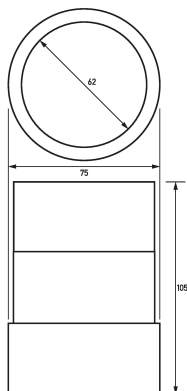
Dibujo acotado Vista de grupos
