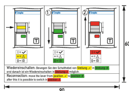
Dibujo acotado Etiqueta de advertencia HAS DFS
