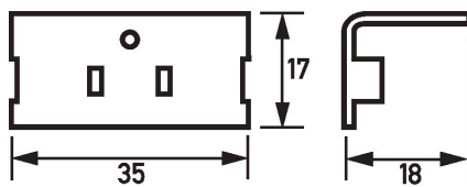
Maßzeichnung KA/RH-KA/KA-DMS (Gruppenansicht)
