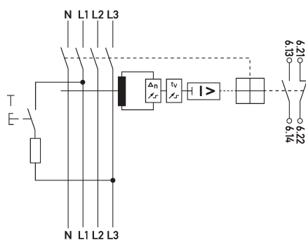
Esquema de conexiones DFL 8 A X
