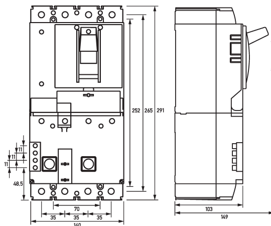
Dibujo acotado DFL 8 A X (Vista de grupos)
