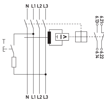
Esquema de conexiones DFL 8 A
