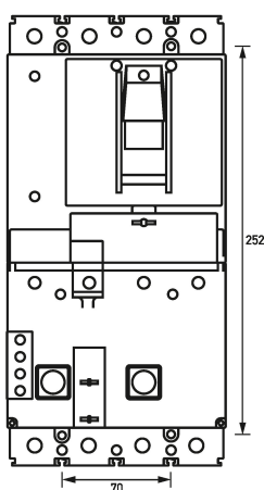
Dibujo acotado Plantilla para taladrar
