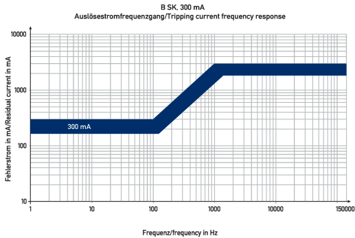
Curva característica B SK 300 mA
