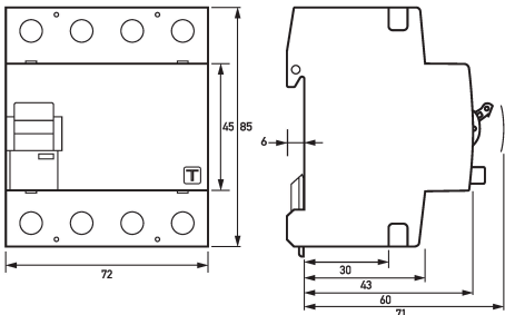
Maßzeichnung Fehlerstromschutzschalter DFS 4 125-4/0,30-B NK S
