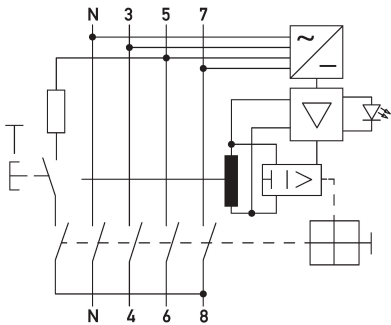
Schaltungsbeispiel Fehlerstromschutzschalter DFS 4 125-4/0,30-B NK S
