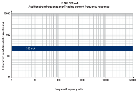
Diagramme Fehlerstromschutzschalter DFS 4 125-4/0,30-B NK S
