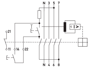
Esquema de conexiones
