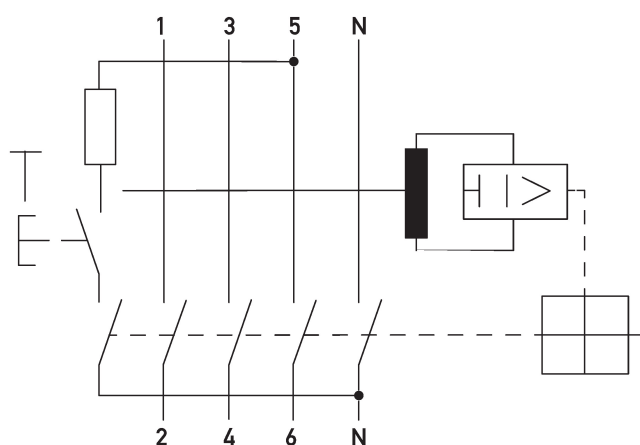
Esquema de conexiones DFS 4 A KV HD, 4 polos N derecha
