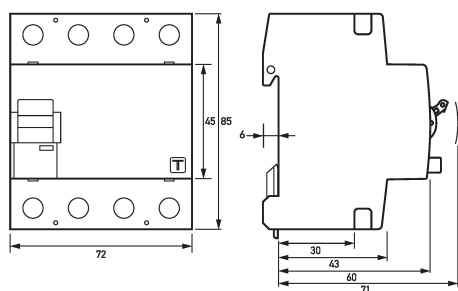
Maßzeichnung Fehlerstromschutzschalter DFS 4 125-4/0,30-A KV R HD
