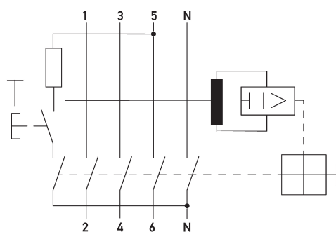
Ejemplo de cableado Interruptores diferenciales DFS 4 125-4/0,30-A R HD
