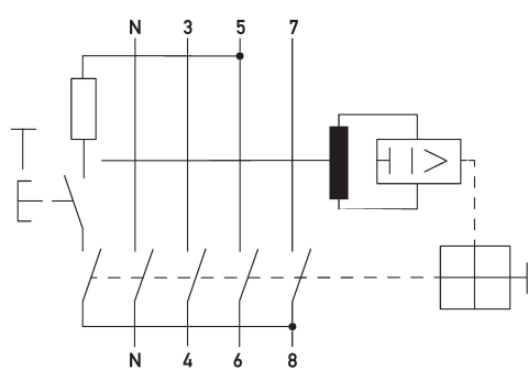
Ejemplo de cableado Interruptores diferenciales DFS 4 AC S, 4 polos
