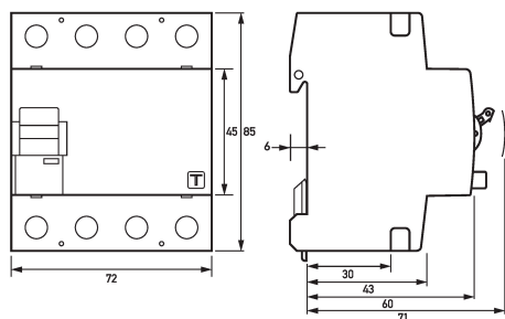
Dibujo acotado Interruptores diferenciales DFS 4 AC S, 4 polos
