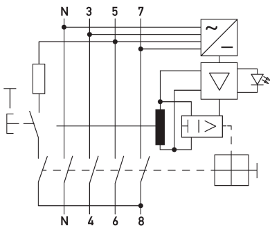
Ejemplo de cableado Interruptores diferenciales DFS 4 125-4/0,10-B NK
