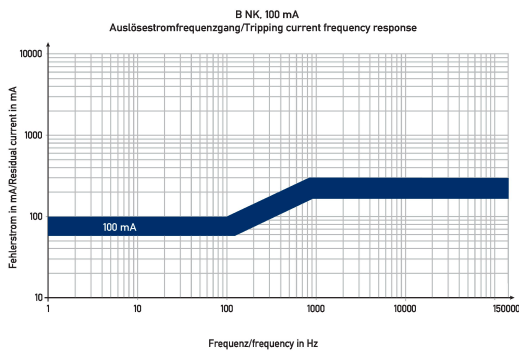
Diagramas Interruptores diferenciales DFS 4 125-4/0,10-B NK
