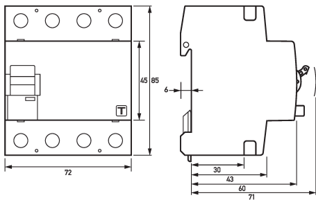
Dibujo acotado Interruptores diferenciales DFS 4 125-4/0,10-B NK
