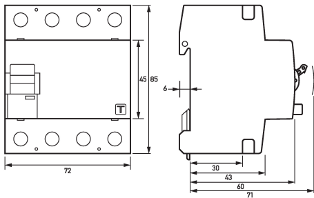
Dibujo acotado Vista de grupos
