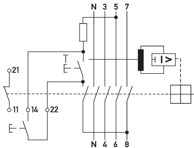
Esquema de conexiones DFS 4 A FT, 4 polos
