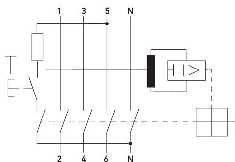
Ejemplo de cableado Interruptores diferenciales DFS 4 125-4/0,03-A R HD
