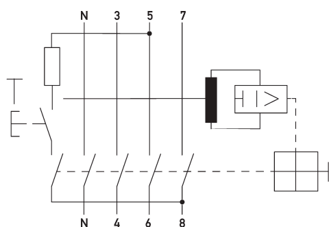
Ejemplo de cableado Interruptores diferenciales DFS 4 125-4/0,03-A HD
