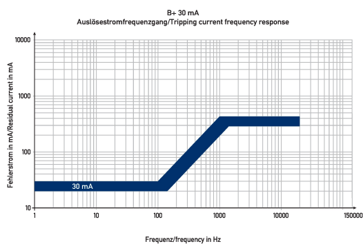
Diagramme Fehlerstromschutzschalter DFS 4 125-4/0,03-B+
