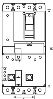
Dibujo acotado Vista de grupos
