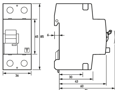
Maßzeichnung Fehlerstromschutzschalter DFS 2 125-2/0,03-A V110
