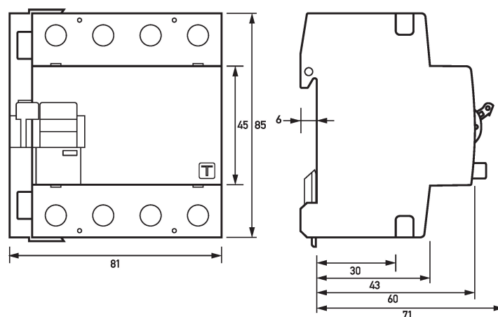
Dibujo acotado DFS 4 A FT, 4 polos (Vista de grupos)
