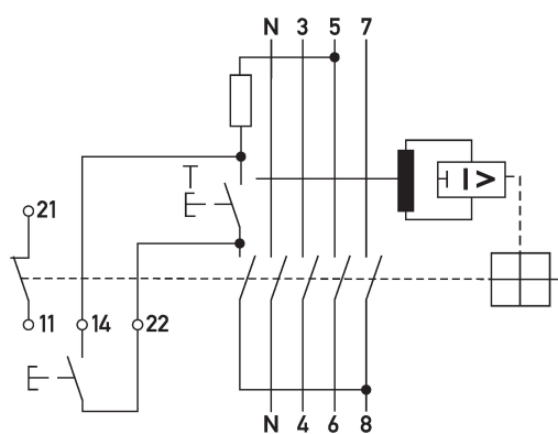
Esquema de conexiones DFS 4 A FT, 4 polos
