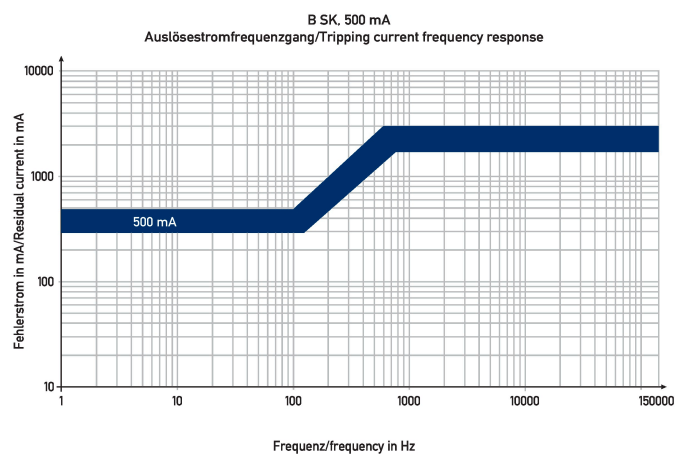
Curva característica B SK 500 mA
