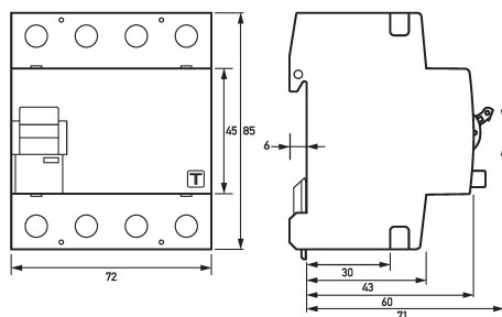
Dibujo acotado Interruptores diferenciales DFS 4 100-4/0,30-A R HD
