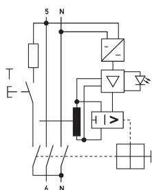
Schaltungsbeispiel Fehlerstromschutzschalter DFS 4 100-2/0,30-B+
