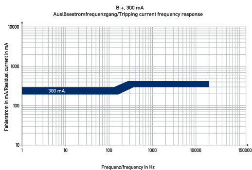
Diagramme Fehlerstromschutzschalter DFS 4 100-2/0,30-B+
