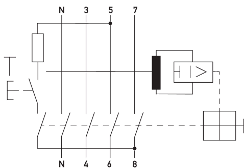
Schaltungsbeispiel Fehlerstromschutzschalter DFS 4 100-4/0,10-A HD
