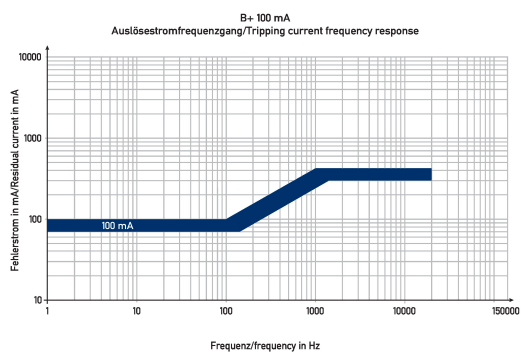
Diagramme Fehlerstromschutzschalter DFS 4 100-4/0,10-B+
