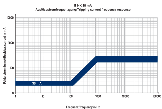
Diagramme Fehlerstromschutzschalter DFS 4 100-4/0,03-B NK HD
