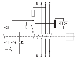
Anschlussschema
