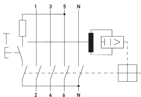
Ejemplo de cableado Interruptores diferenciales DFS 4 100-4/0,03-A KV R
