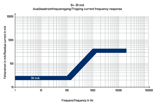
Diagramme Fehlerstromschutzschalter DFS 4 100-2/0,03-B+
