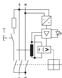
Schaltungsbeispiel Fehlerstromschutzschalter DFS 4 100-2/0,03-B+
