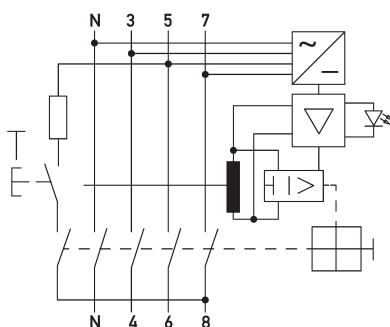
Schaltungsbeispiel Fehlerstromschutzschalter DFS 4 080-4/0,50-B SK S
