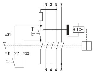
Anschlussschema
