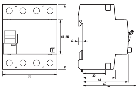
Maßzeichnung Fehlerstromschutzschalter DFS 4 080-4/0,50-A
